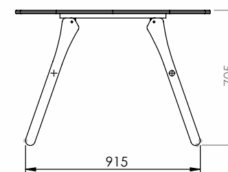
1. stół wysoki-rozłożony
